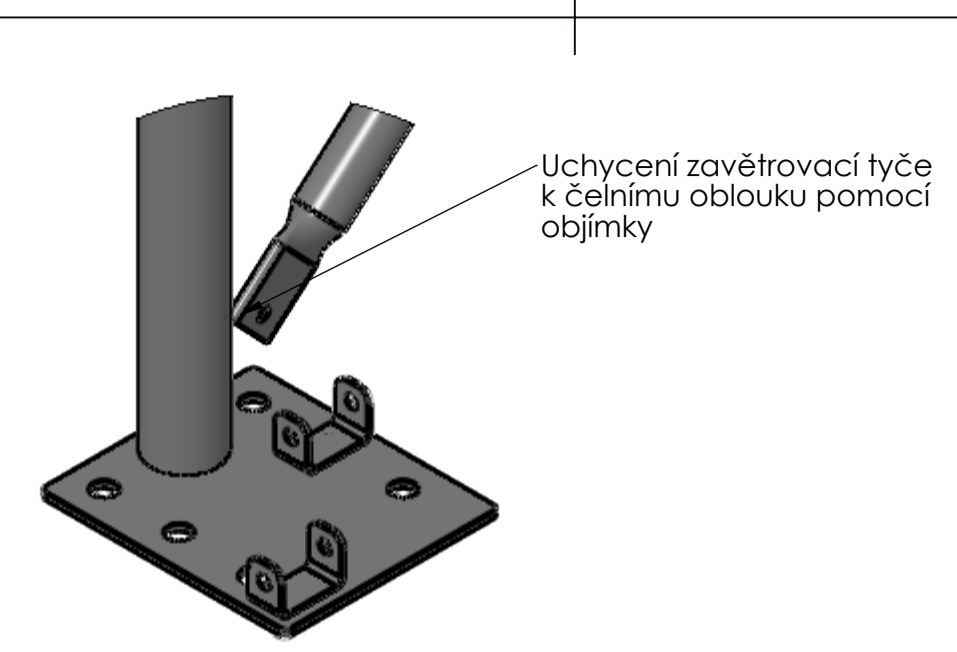
DETAIL A MĚŘITKO 1 : 5
